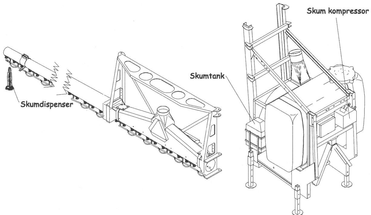
Skematisk placering af dispenser, skumtank og kompressor
